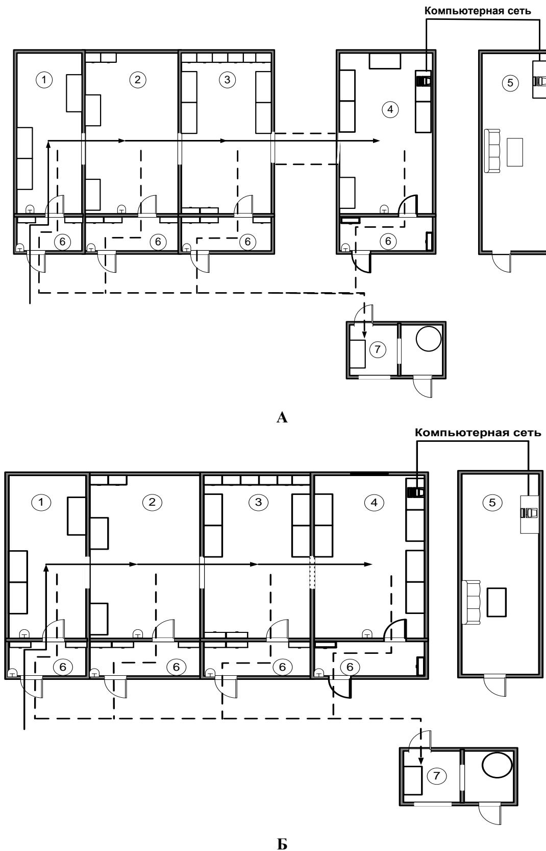
Рис.1. Рекомендуемые схемы размещения помещений (рабочих зон) лаборатории, использующей МАНК с электрофоретической и (или) гибридно-ферментативной детекцией продуктов амплификации (А и Б).
